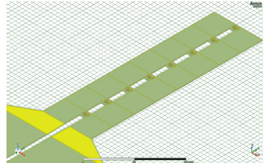
Figure 1 : Exemple de réseau linéaire de photodiodes. Modélisation électromagnétique par méthode des éléments finis à l'aide du logiciel Ansys HFSS.
