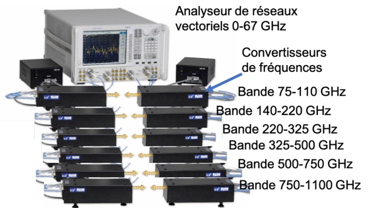
Figure 1. Problématique de la mesure large bande en gamme millimétrique et THz. Analyseur de réseaux vectoriel et extensions nécessaires (convertisseurs de fréquences) pour couvrir la bande 0-1 THz. Il faut 6 systèmes d’extension en plus de l’analyseur de réseau basse fréquence. Coût total (~1M€). Un seul convertisseur est utilisable à la fois entraînant de multiples opérations manuelles et procédures de calibration. (Adaptée de vadiodes.com)
